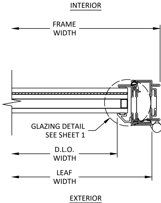
F 6 HORIZONTAL SECTION HINGE JAMB
